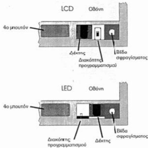
Σχίμα 4. Ο διακόπτης προγραμματισμού
